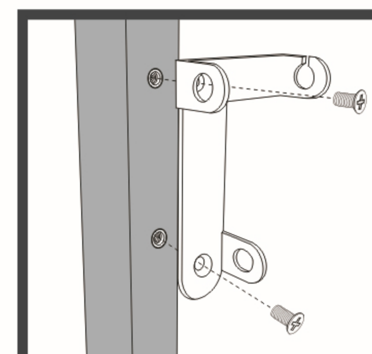
СЮРМЕ ЗА ДВУКРИЛА ВРАТА ГОРНО
