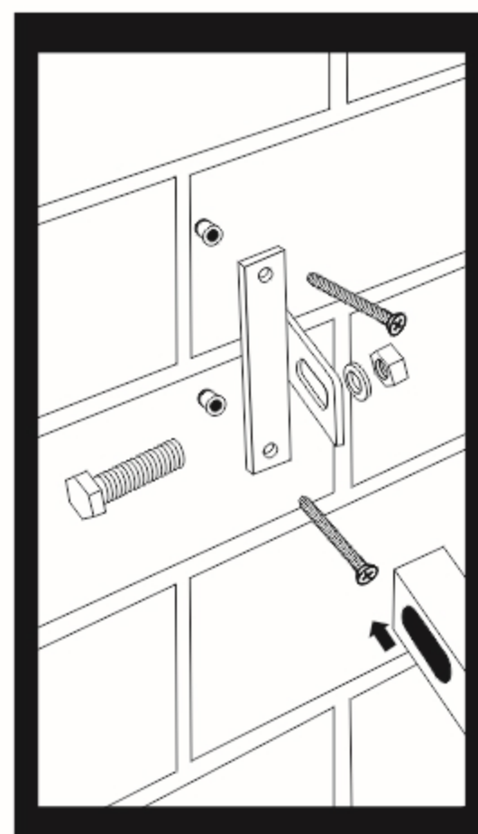
ФИКСАТОР ЗА ОГРАДНО ПАНО ТИП Т
