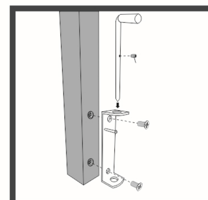
СЮРМЕ ЗА ДВУКРИЛА ВРАТА ДОЛНО
